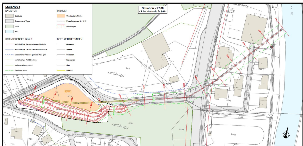
Abb. 21: BUD: Gemeinde Dittingen / Stadt Laufen Gewässerraum Schachletebach – VORPROJEKT vom 22.03.2023
